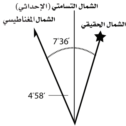
الشمال الحقيقي والشمال التسمتي والشمال المغناطيسي
