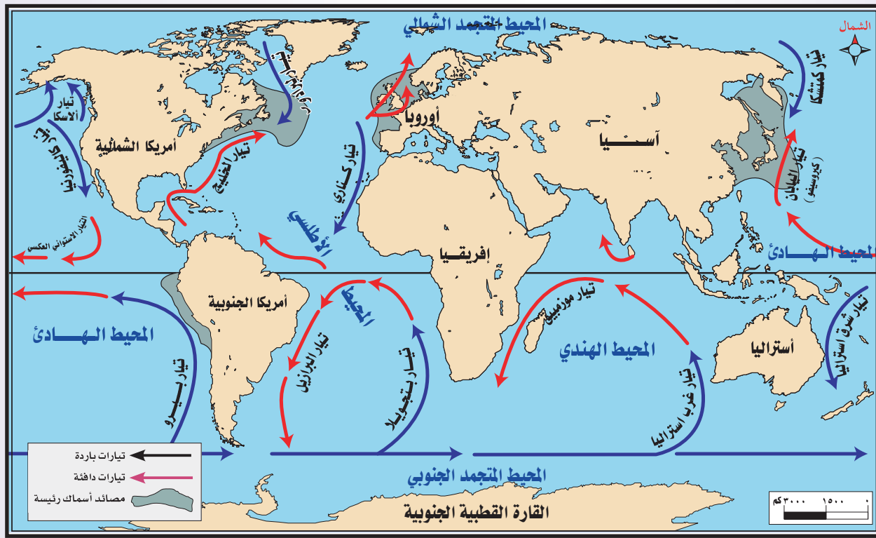
التيارات المحيطية في العالم
