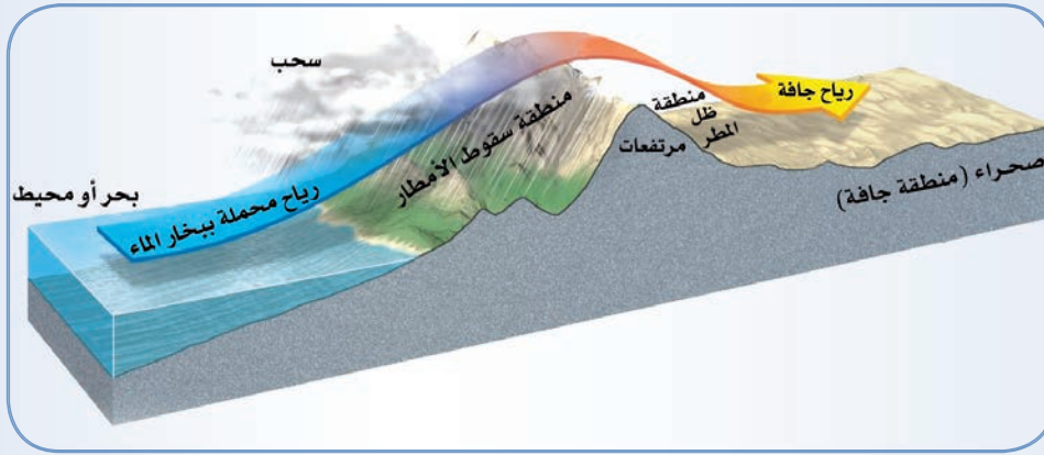
المطر التضاريسي
