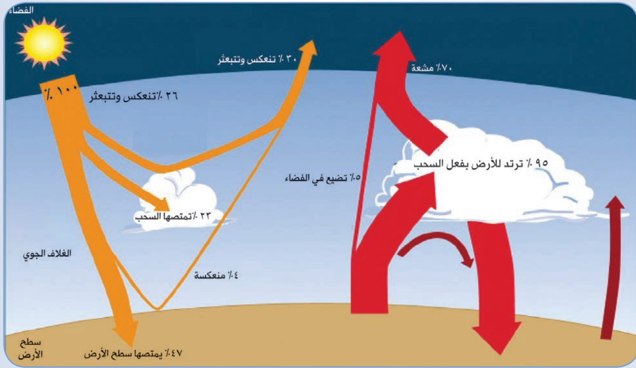
الألبيدو الأرضي
