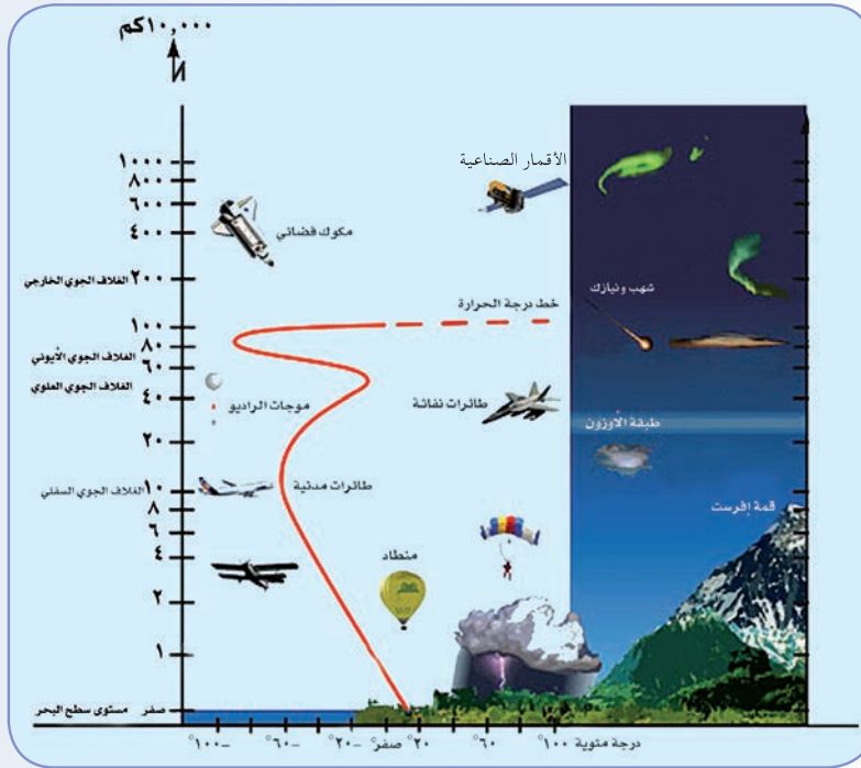
طبقات الغلاف الجوي
