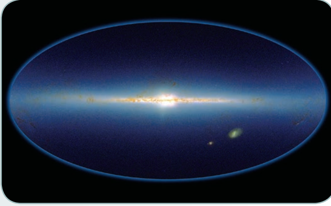
مجرة سكة الثبانة ( منظر جانبي )
