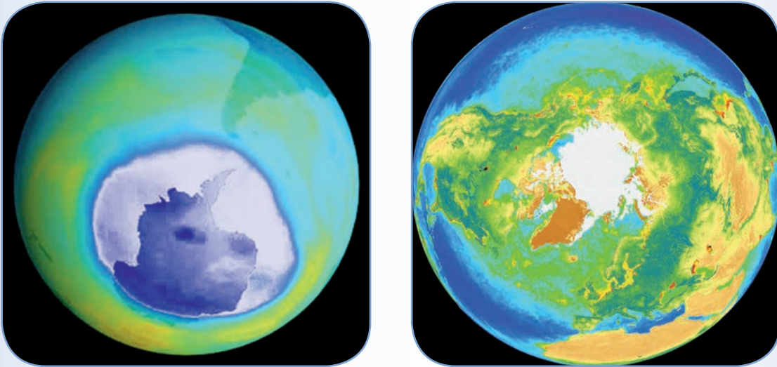
ثقب الأوزون فوق القطبين الشمالي والجنوبي - صورة للكرة الأرضية بالأقمار الصناعية
