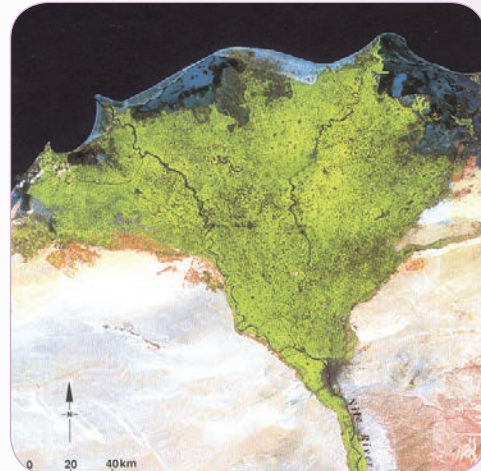
دلتا نهر النيل
