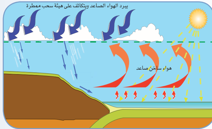
المطر التصاعدي
