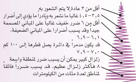
الزلازل وكيفية قياسها
