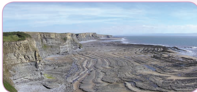
تعرية بحرية
