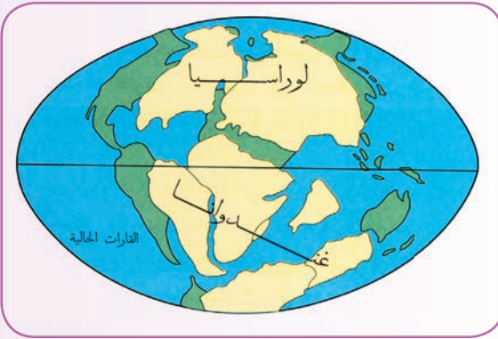
لوراسيا - غندوانا
