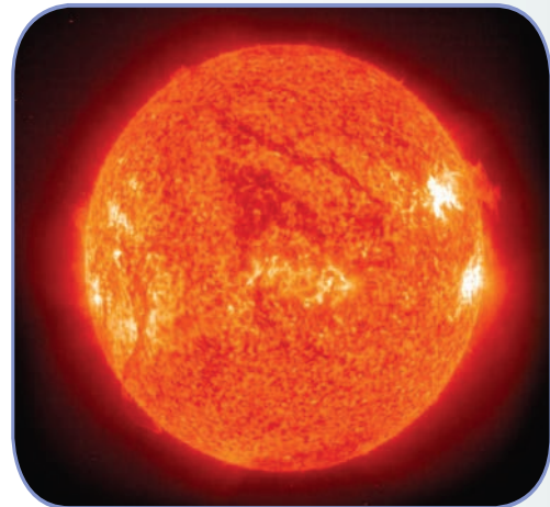
الشمس
