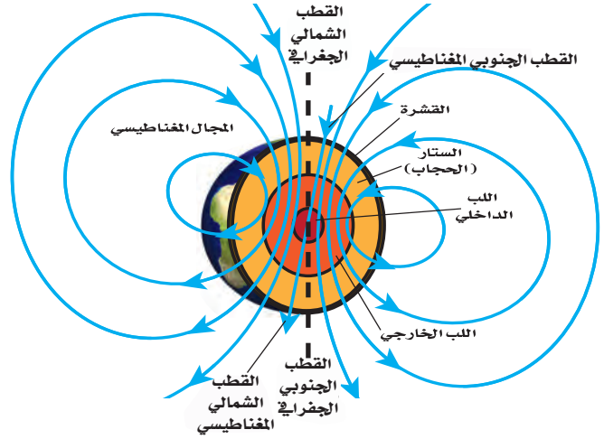
الشكل ٦ للأرض مجال مغناطيسي مشابه للمجال المتكون حول قضيب المغناطيس. ويعد القطب الشمالي الجغرافي للأرض جنوباً مغناطيسياً كما يعد القطب الجنوبي الجغرافي للأرض شمالاً مغناطيسياً.
