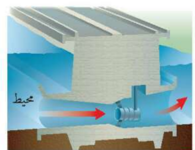
أ خلال المد تدبر حركة الماء التوربين المرتبط مع المولد الكهربائي، وعند اكتمال المد تغلق البوابة لتحتجز الماء خلف السد.
