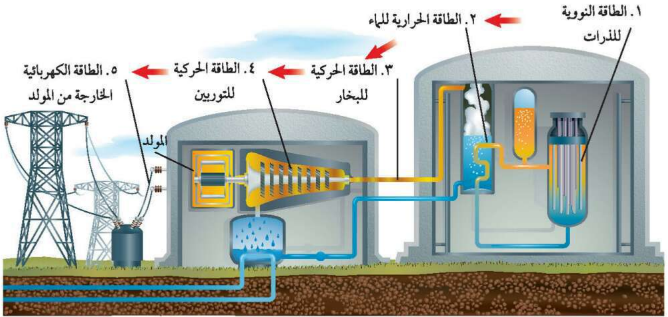
الشكل ٧ تحدث سلسلة من تحولات الطاقة للحصول على الطاقة الكهربائية من الطاقة النووية. صف. كيف تنتج الحرارة خلال التفاعلات النووية؟
