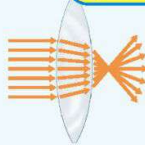
عدسة محدبة
