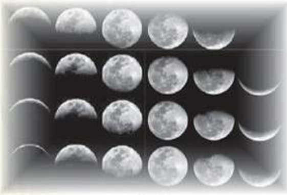
منازل القمر
