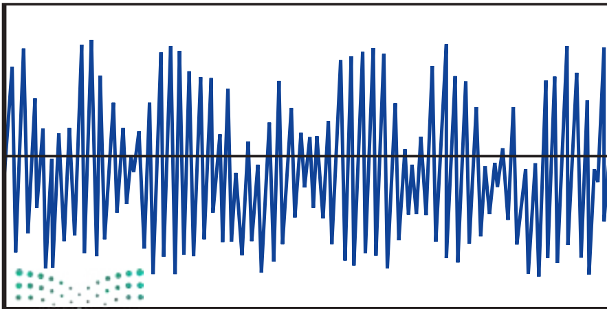
■ الشكل 8-16 يتكون الضجيج من ترددات متعددة، ويتضمن تغيرات عشوائية في التردد والسعة.
