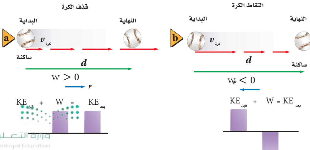
الشكل 2-4 الطاقة الحركية بعد قذف الكرة أو التقاطها تساوي الطاقة الحركية قبل عملية القذف أو الالتقاط + الشغل المبذول.
