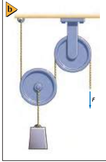
■ الشكل 10-3 الفائدة الميكانيكية
