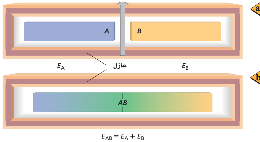
■ الشكل 5-8 نظام مكون من نموذجين لقالبين عند درجات حرارة مختلفة، وهما مفصولان في الحالة الابتدائية (a). وعندما يتلامس القالبان فإن الحرارة تتدفق من القالب الساخن إلى القالب الأبرد (b). وتبقى الطاقة الكلية ثابتة.
