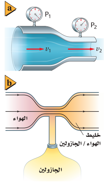
■ الشكل 6-16 يكون الضغط P_1 أكبر من P_2 ؛ لأن v_1 أقل من v_2 (a). يعمل الضغط المنخفض في الجزء الضيق من أنبوب المازج (carburetor) على سحب الوقود إلى مجرى الهواء (b).
