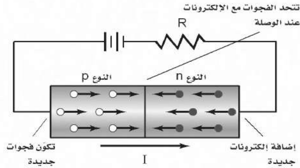
الدايدود المتحاز أمامياً
