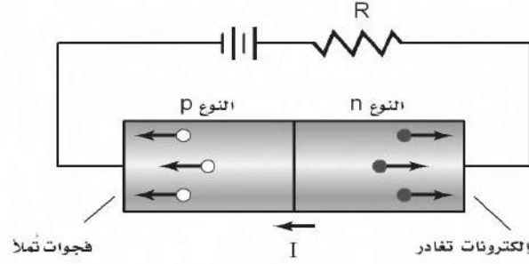
الدايدود المتحاز عكسياً
