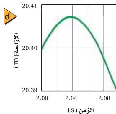
■ الشكل 15-3 في نظام إحداثي اتجاهه الموجب إلى أعلى: a و b تتناقص سرعة الكرة المقذوفة إلى أعلى حتى تصبح صفراً بعد زمن 2.04 s ثم تزايد سرعتها في الاتجاه السالب في أثناء سقوطها. c و d يُظهر الرسمان البيانيان لمنحنى (الإزاحة - الزمن) ارتفاع الكرة في فترات زمنية مماثلة.
