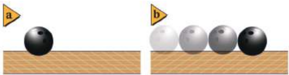
■ الشكل 4-6 الكرة الساكنة تبقى ساكنة (a) الكرة المتدحرجة بسرعة ثابتة وعلى خط مستقيم تبقى على درجتها دون توقف ما لم تؤثر عليها قوى خارجية (b).
