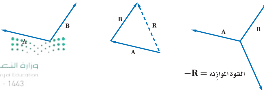
■ الشكل 12-5 للقوة الموازنة مقدار القوة المحصلة نفسها، ولكنها تعاكسها في الاتجاه.
