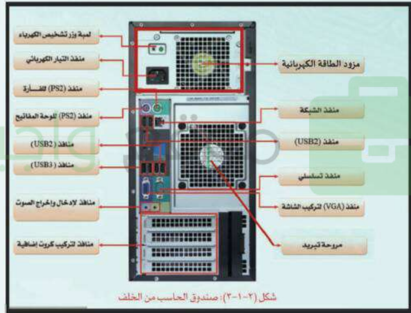
شكل (٣-١-٢): صندوق الحاسب من الخلف
