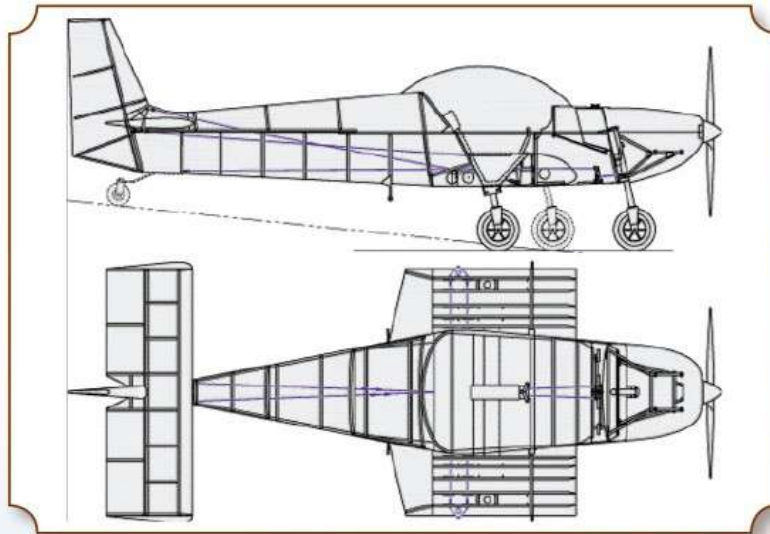
شكل (٦) تصميم.
