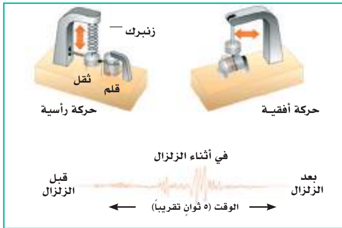
طريقة عمل السيسموغراف
